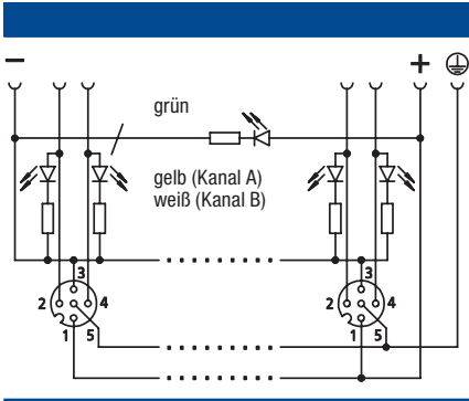
Schaltbild ASBV-R... LED
