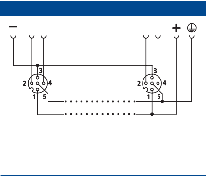
Schaltbild ASBV-R...
