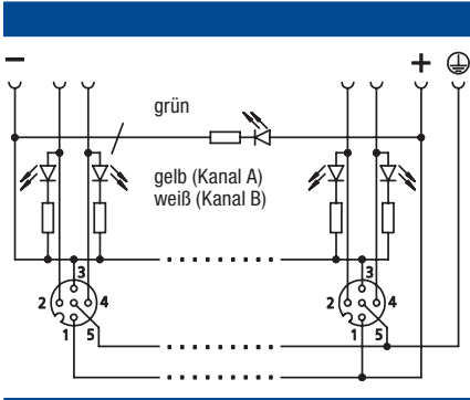
Schaltbild ASBSV-R... LED
