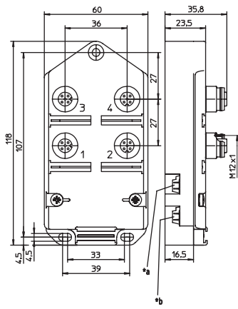
0911 ANC 403 *a = AS-Interface Standard-Flachkabel *b = Zusatz-Spannungsversorgung (AS-Interface Ausgangsstufen)
