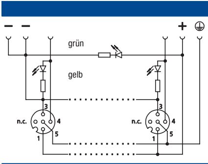
Schaltbild ASB-R... LED
