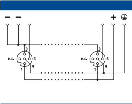
Schaltbild ASBS-R...
