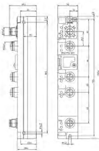
0940 PSL 601 | 0940 PSL 602 | 0940 PSL 603
