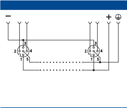
Schaltbild ASBSV-R...
