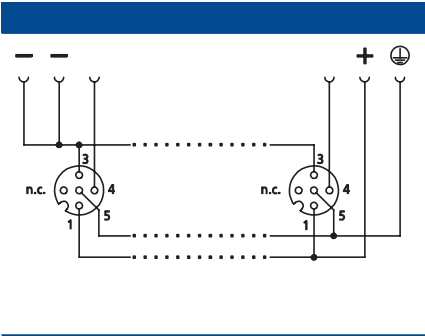
Schaltbild ASB-R...
