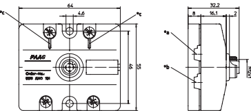
0911 ANC 101 *a = LINE 1: Standardflachkabel *b = LINE 2: Zusatz-Spannungsversorgung *c = Erdungsfeder
