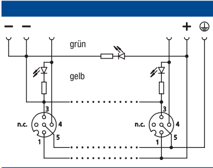
Schaltbild ASBS-R... LED
