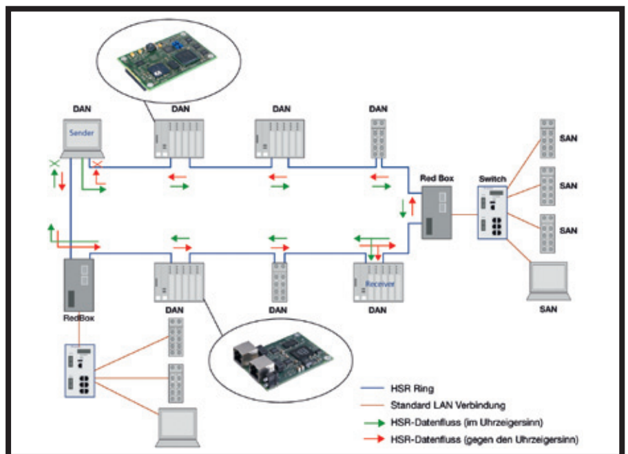
Abb. 4 Eine Kombination aus Stand-alone und Embedded Switches ist eine optimale Konfiguration für industrielle Umgebungen.
