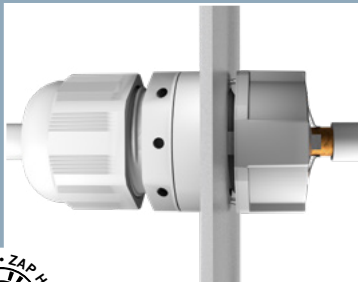
MagikNUT mit VentGLAND® IP68 / 69 Kabelverschraubung aus Kunststoff.
