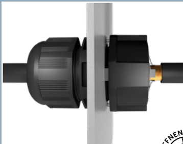
MagikNUT mit ESKV IP68 / 69 Kabelverschraubung aus Kunststoff.
