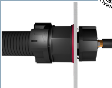
MagikNUT mit Kunststoff IP68 Wellrohr- verschraubung BraceFITTING und dem Kunststoff-Wellrohr BraceCONDUIT.
